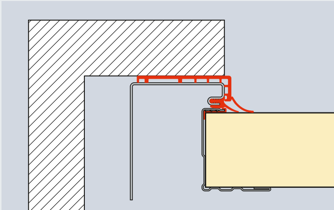
Battuta laterale con equipaggiamento ThermoFrame
